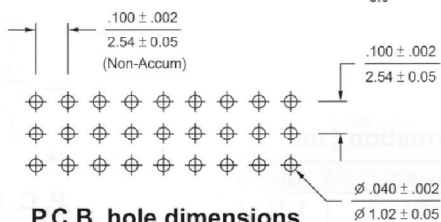
P.C.B. hole dimensions
